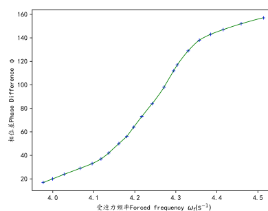
图 10: 阻尼 4 相位差与频率曲线图
