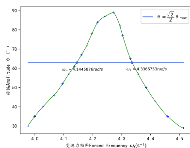
图 9: 阻尼 4 振幅与频率曲线图
