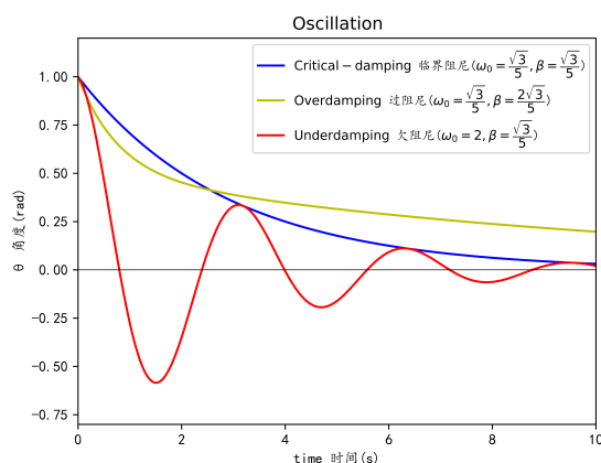
图 2: 不同阻尼系数下的振动曲线 \theta(t)
