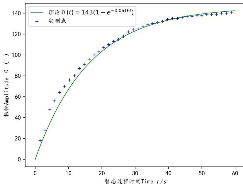
图 13: 受迫振动中暂态振幅与时间曲线图 (阻尼 2)
