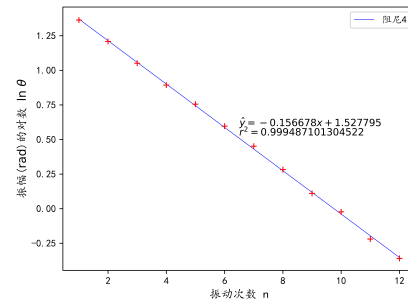
图 6: 阻尼 4 振幅随振动次数曲线图
