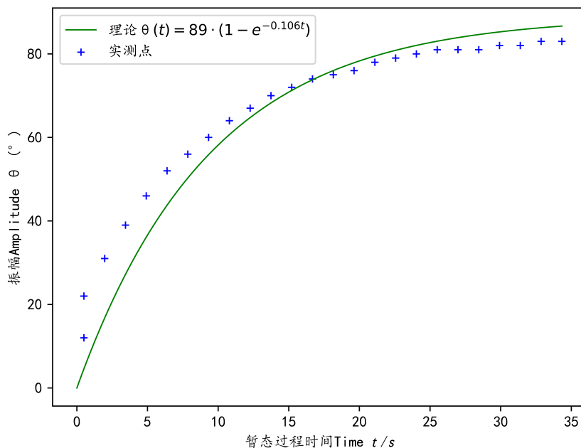
图 14: 受迫振动中暂态振幅与时间曲线图 (阻尼 4)
