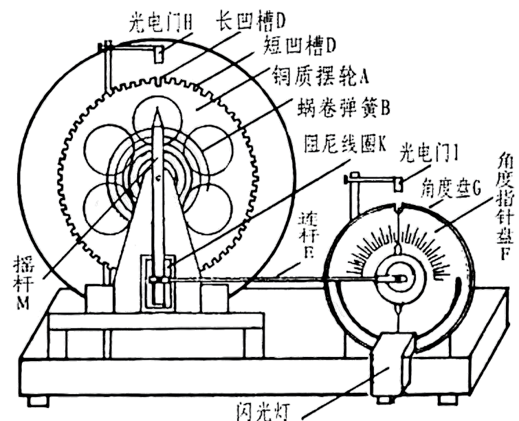
图 3: 波尔共振仪结构示意图
