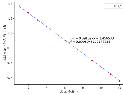
图 5: 阻尼 2 振幅随振动次数曲线图
