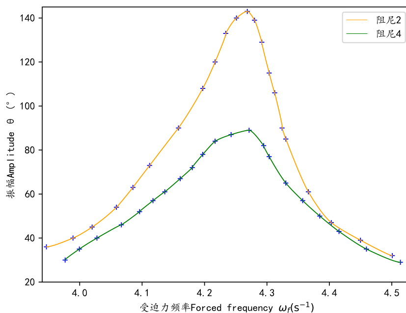
图 11: 不同阻尼系数下受迫振动振幅与强迫力频率关系图
