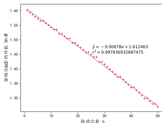
图 4: 零阻尼下振幅对数和振动次数关系图
