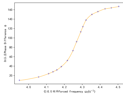
图 8: 阻尼 2 相位差与频率曲线图
