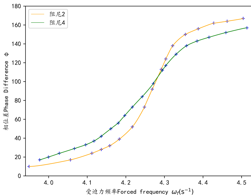
图 12: 不同阻尼系数下受迫振动相位差与强迫力频率关系图
