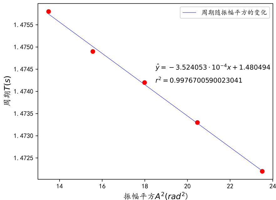
图 15: 无阻尼周期随振幅平方变化拟合直线
