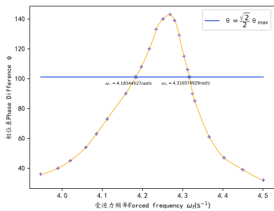
图 7: 阻尼 2 振幅与频率曲线图
